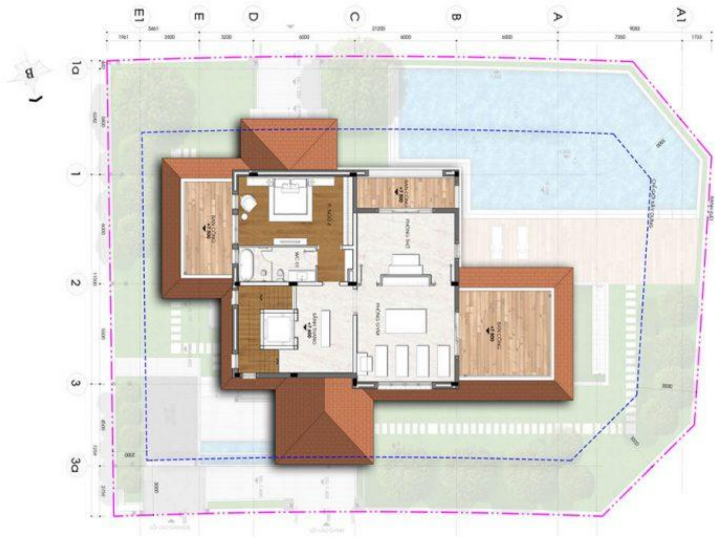
Mặt bằng Tầng 3 Villa 23-L3f
